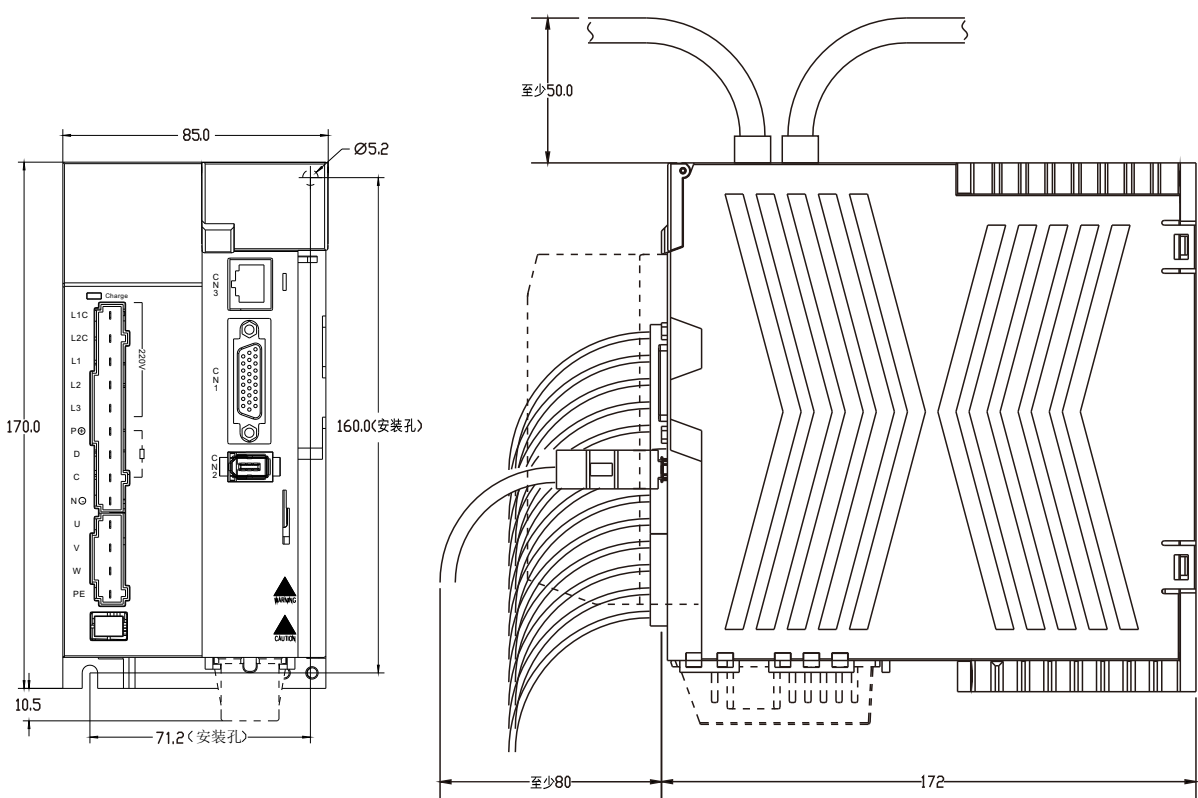
380V 50A/75A 驱动器外形尺寸
