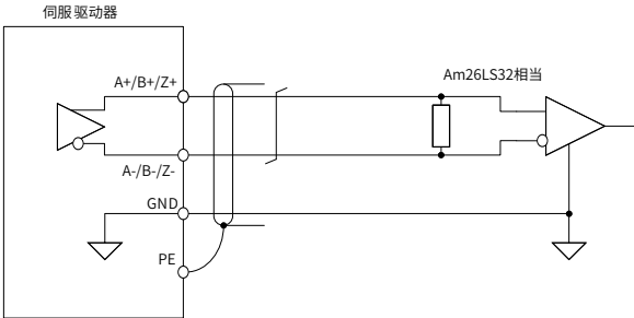
差分脉冲输出:
