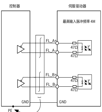
COMM2差分输入方式
