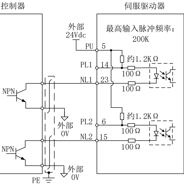
脉冲输入接线，漏型方式，外部电源
