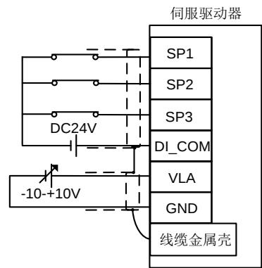
注：模拟量速度限制（VLA）
