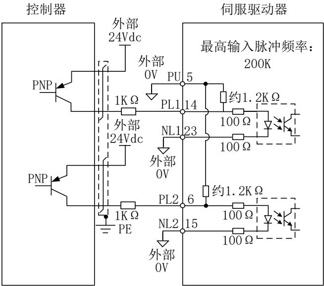
脉冲输入接线，源型方式，外部电源
