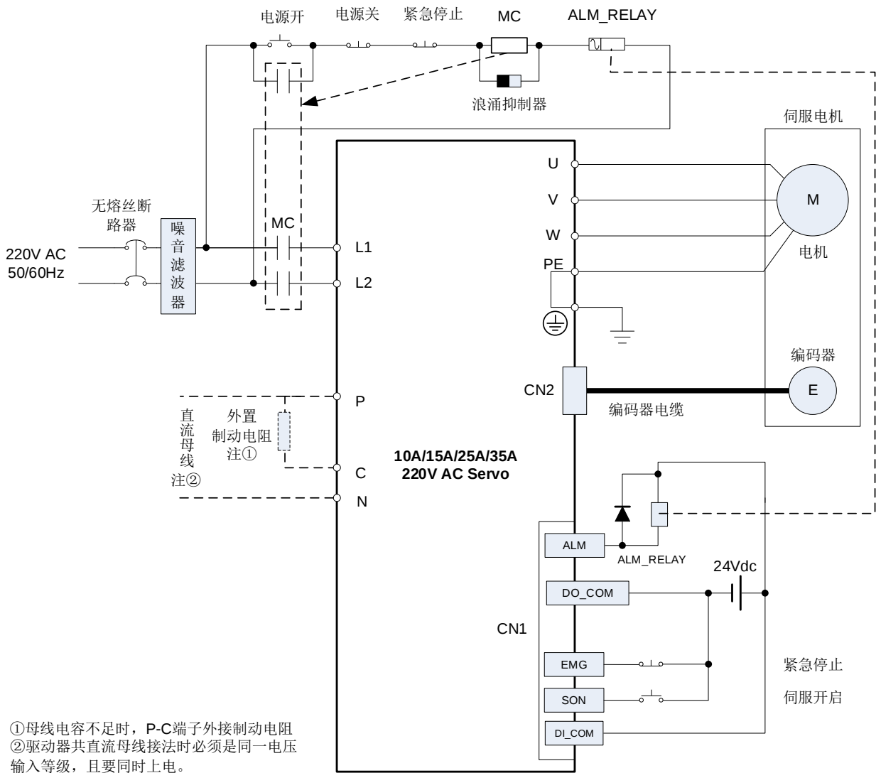
使用单相 AC 220V 电源的接线图
