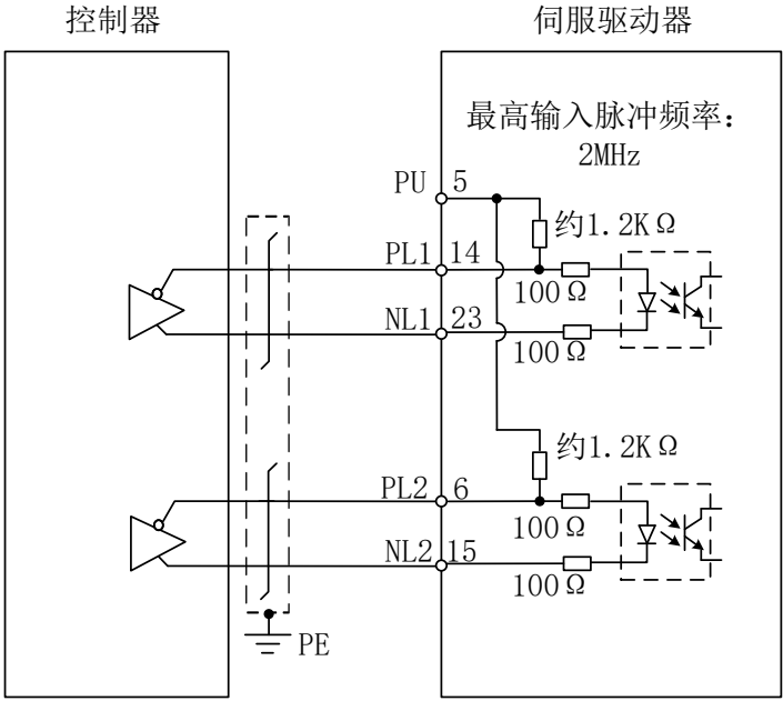
差分位置输入接线
