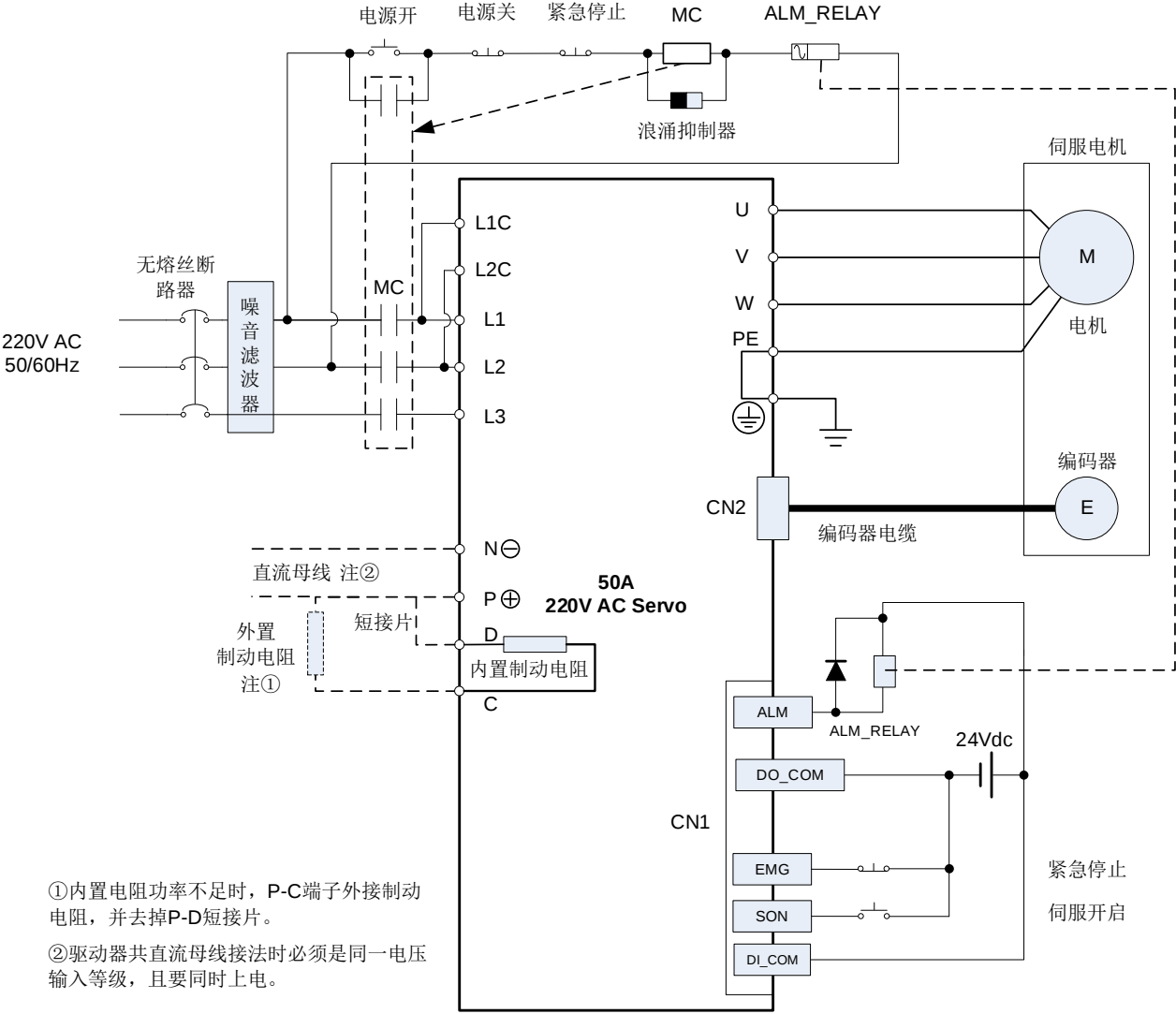
使用三相 AC 220V 电源的接线图
