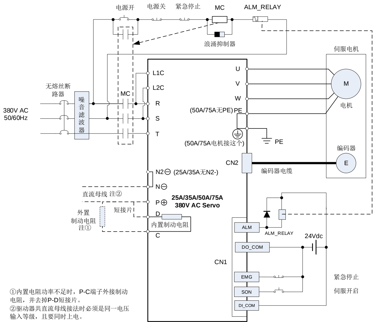
使用三相 AC 380V 电源的接线图
